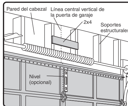
MONTAJE DE TECHO OPCIONAL PARA EL SOPORTE DEL CABEZAL
